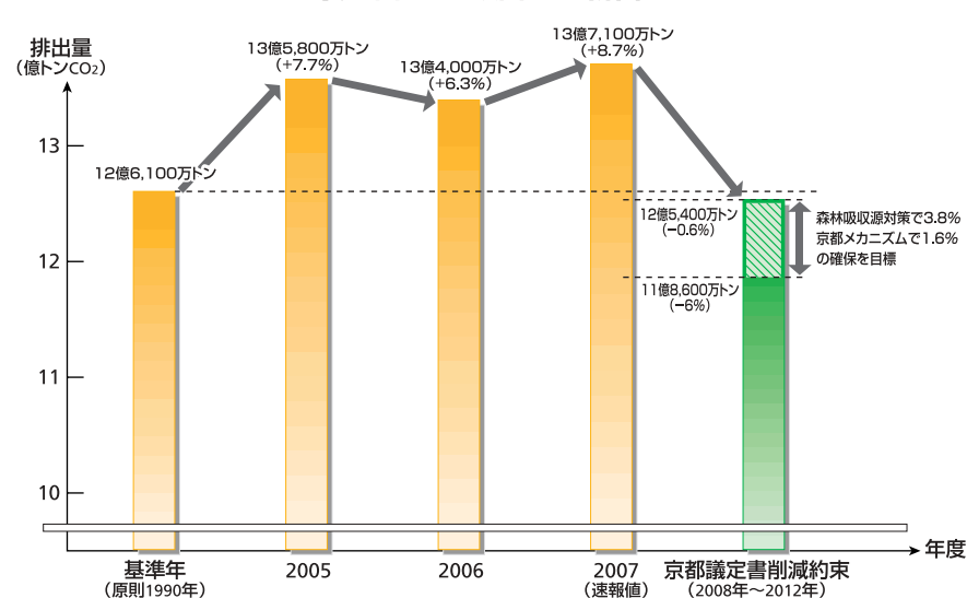
我が国の温室効果ガス排出量
