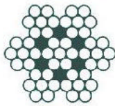
7 x 7 + 0 DIN 3055 (AISI 316)
