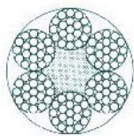
6 x 19 + 1 DIN 3060
