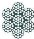
7 x 19 + 0 DIN 3060 (AISI 316)
