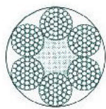
6 x 37 + 1 DIN 3066
