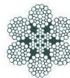
6 x 36 + 0 WS DIN 3064
