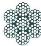
7 x 19 + 0 DIN 3060
