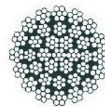
35 x 7 + 0 DIN 3071
