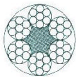
6 x 7 + 1 DIN 3055
