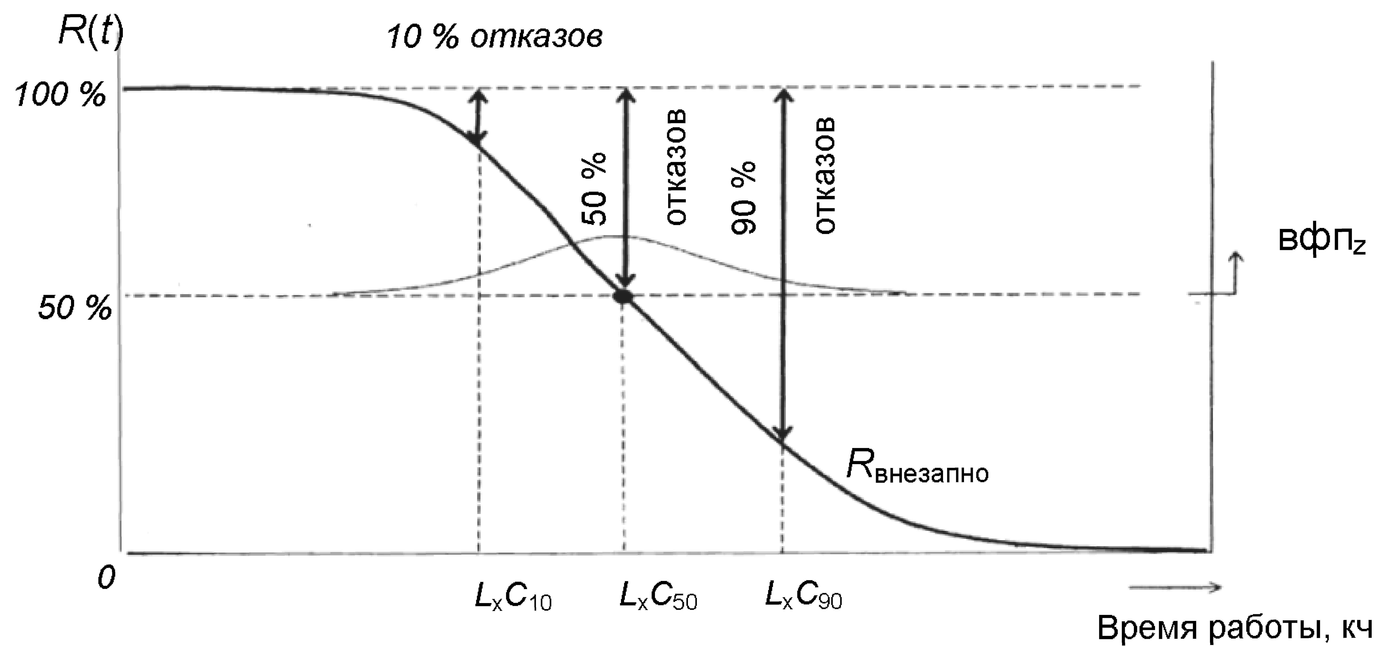
Рисунок С.4 – Кривая надежности внезапного прекращения свечения R_{внезапно}
