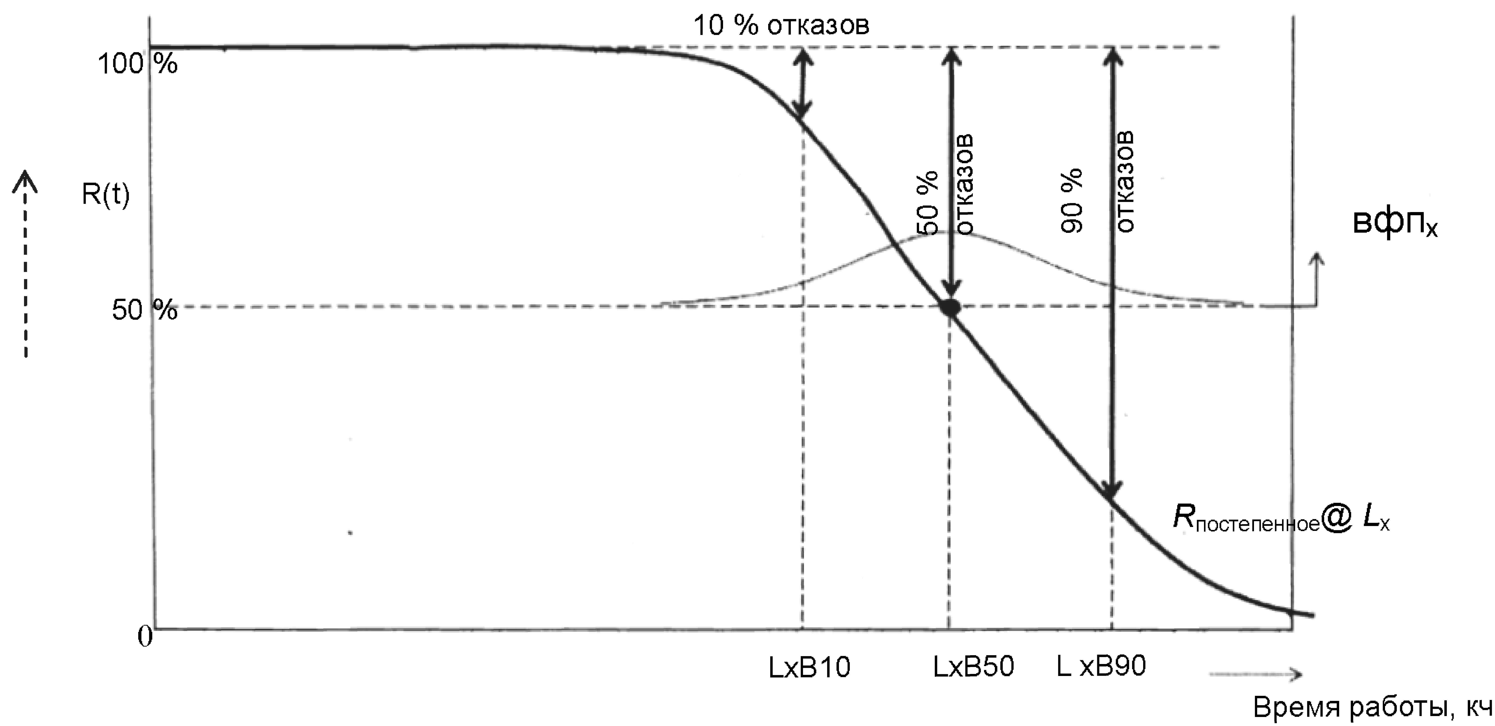
Рисунок С.3 – Кривая надежности постепенного снижения светового потока R_{постепенное}
