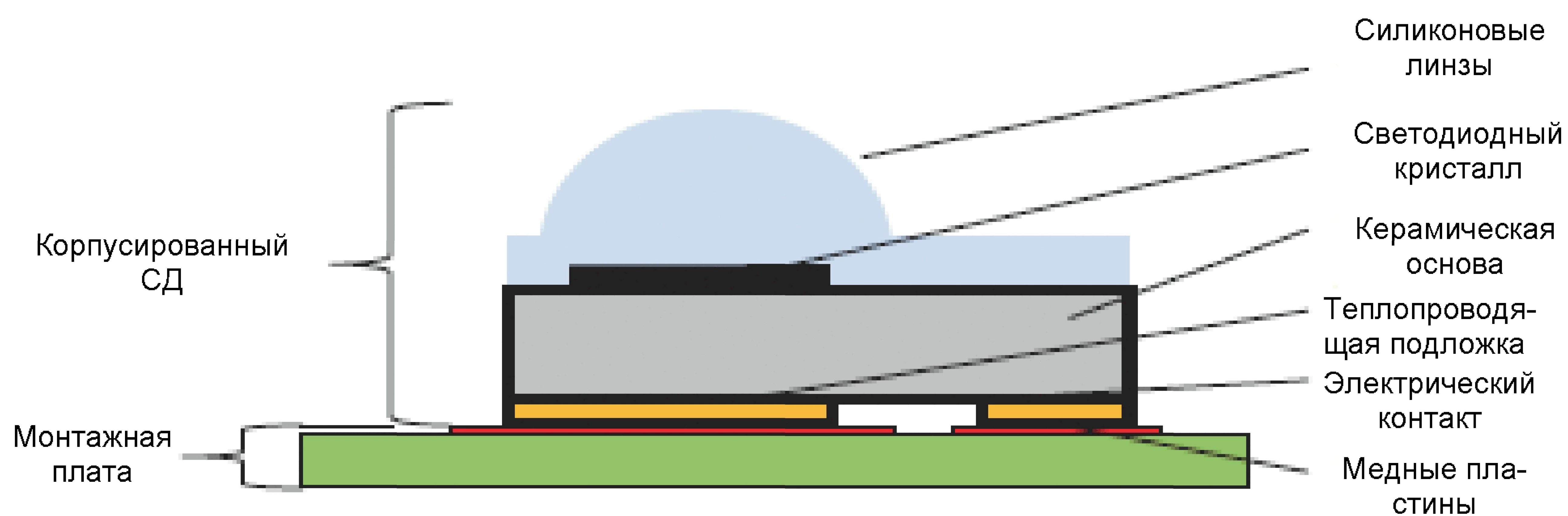
б) Поверхностный монтаж корпусированного СД без выводов
