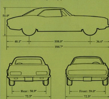
INTERIOR DIMENSIONS (sport coupe)
