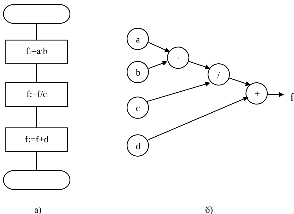
Рис. 1. 1. Процедурное (а) и потоковое (б) представление алгоритма вычисления значения f = ab/c + d
