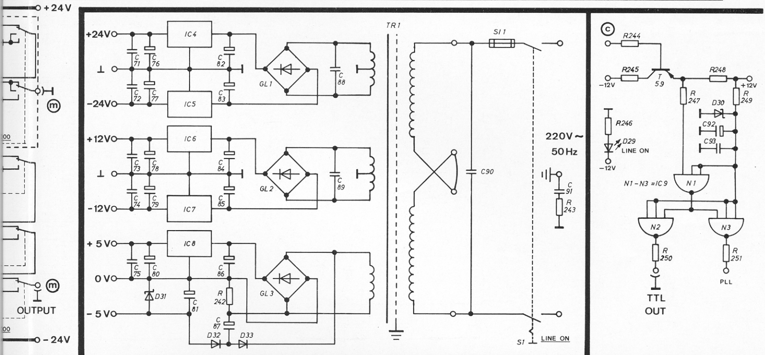
Stromlaufplan Hauptplatine
