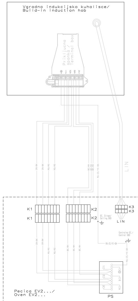
Prikaz vezave - pogled od spodaj / Connection layout - bottom view
