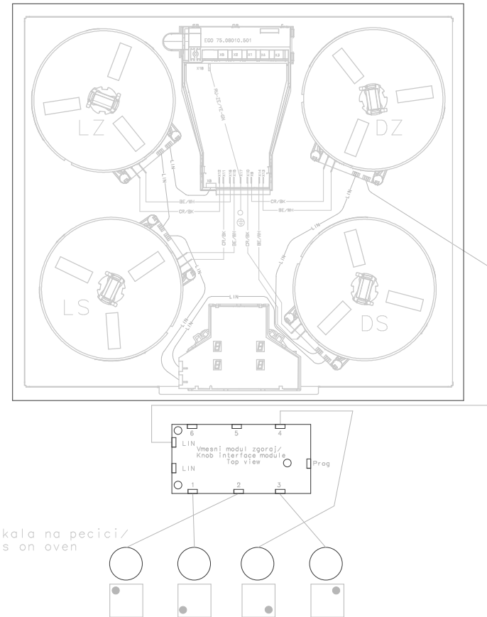
Indukcijsko kuhališče - pogled notranjost od zgoraj / Induction hob - inside top view
