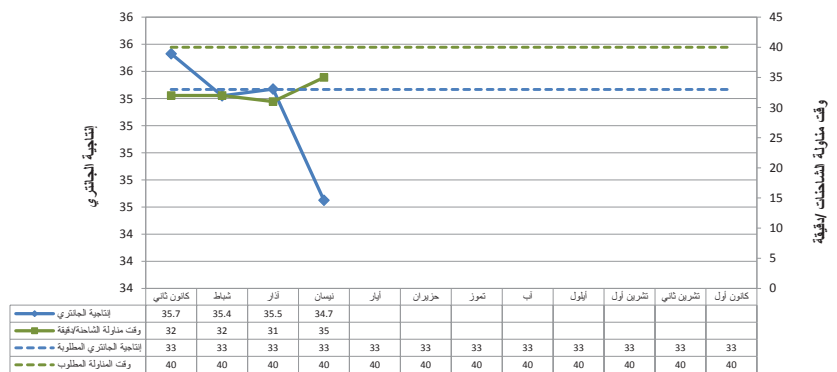
إنتاجية الجانترى ووقت مناولة الشاحنات
