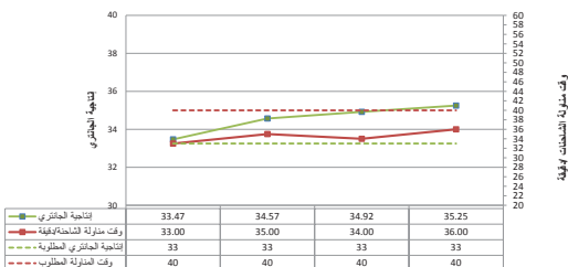
إنتاجية الجانترى ووقت مناولة الشاحنات / حسب الشفت
