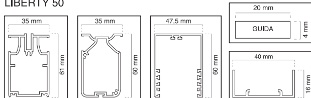
LIBERTY 50
