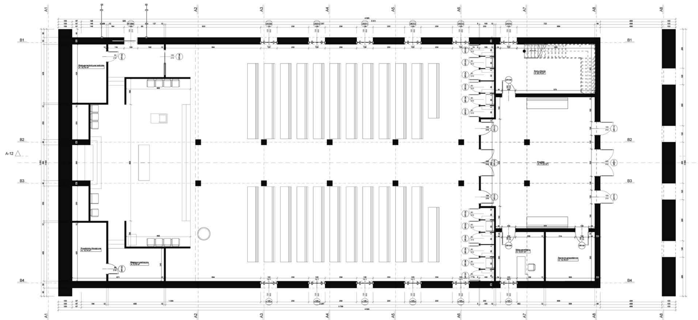
RZUT PARTERU KOŚCIOŁA
