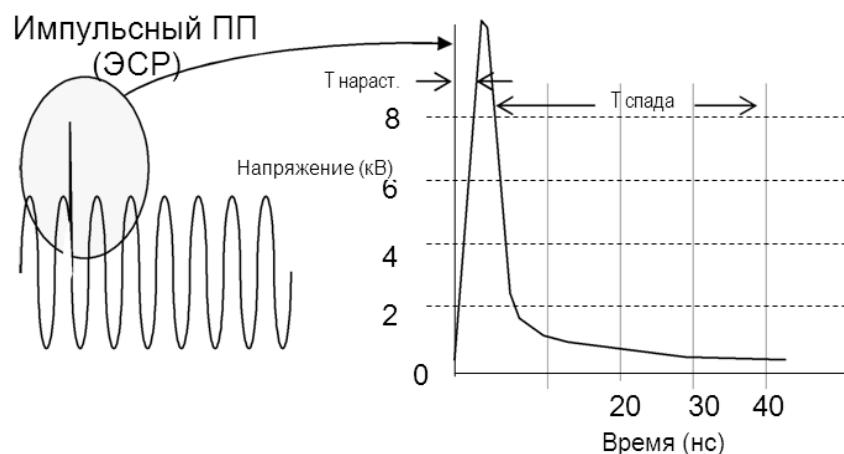
Рисунок 3. – Импульсный переходный процесс.
