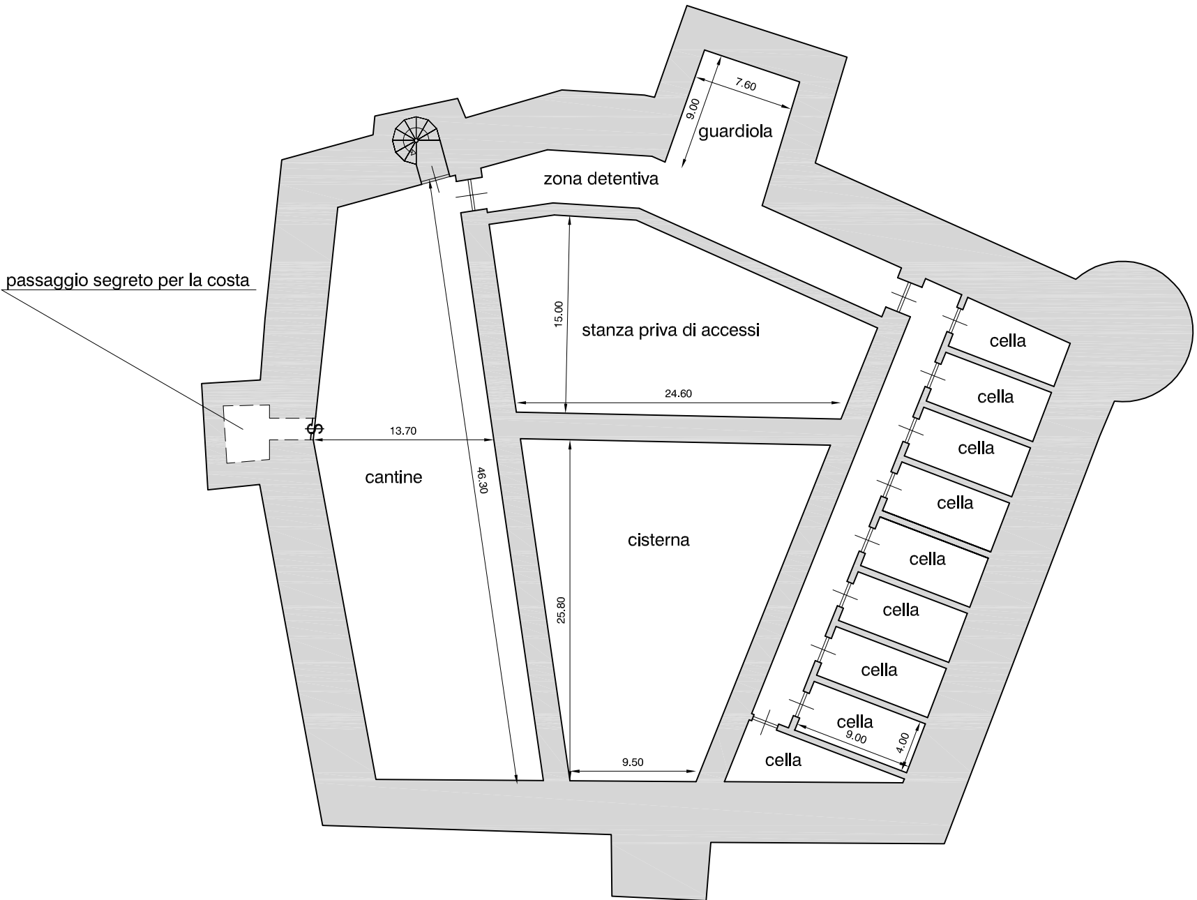
PIANTA PIANO SOTTERRANEO
