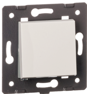
MODUL IZMJENIČNI PREKIDAČ KATALOŠKI BROJ 1FKSBIG-61 DIMENZIJE: 45x45x35 mm Radni napon: izmjenična struja 110 V-250 V / 50 Hz-60 Hz Jakost električne struje: 10A
