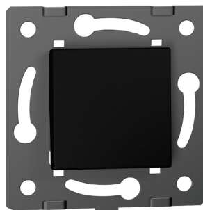
MODUL IZMJENIČNI PREKIDAČ KATALOŠKI BROJ 1FKSBIG-62 DIMENZIJE: 45x45x35 mm Radni napon: izmjenična struja 110 V-250 V / 50 Hz-60 Hz Jakost električne struje: 10A
