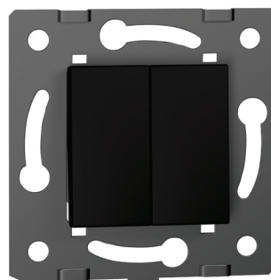
MODUL IZMJENIČNI DVOSTRUKI PREKIDAČ KATALOŠKI BROJ 1FKS-62 DIMENZIJE: 2*modul 22,5mm Radni napon: izmjenična struja 110 V-250 V / 50 Hz-60 Hz Jakost električne struje: 10A
