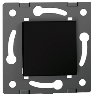
MODUL JEDNOPOLNI PREKIDAČ KATALOŠKI BROJ 1FKBIG-62 DIMENZIJE: 45x45x35 mm Radni napon: izmjenična struja 110 V-250 V / 50 Hz-60 Hz Jakost električne struje: 10A
