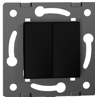
MODUL SERIJSKI PREKIDAČ KATALOŠKI BROJ 1FKS-62 DIMENZIJE: 2*modul 22,5mm Radni napon: izmjenična struja 110 V-250 V / 50 Hz-60 Hz Jakost električne struje: 10A
