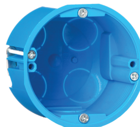
UZIDNA KUTIJA S VIJCIMA PLAVE BOJE KATALOŠKI BROJ PV60D *ZA GIPS UGRADNJU DIMENZIJE: Ø60*60 mm
