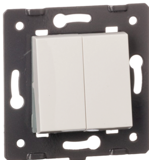
MODUL SERIJSKI PREKIDAČ KATALOŠKI BROJ 1FKS-61 DIMENZIJE: 2*modul 22,5mm Radni napon: izmjenična struja 110 V-250 V / 50 Hz-60 Hz Jakost električne struje: 10A
