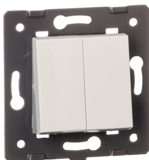
MODUL IZMJENIČNI DVOSTRUKI PREKIDAČ KATALOŠKI BROJ 1FKS-61 DIMENZIJE: 2*modul 22,5mm Radni napon: izmjenična struja 110 V-250 V / 50 Hz-60 Hz Jakost električne struje: 10A
