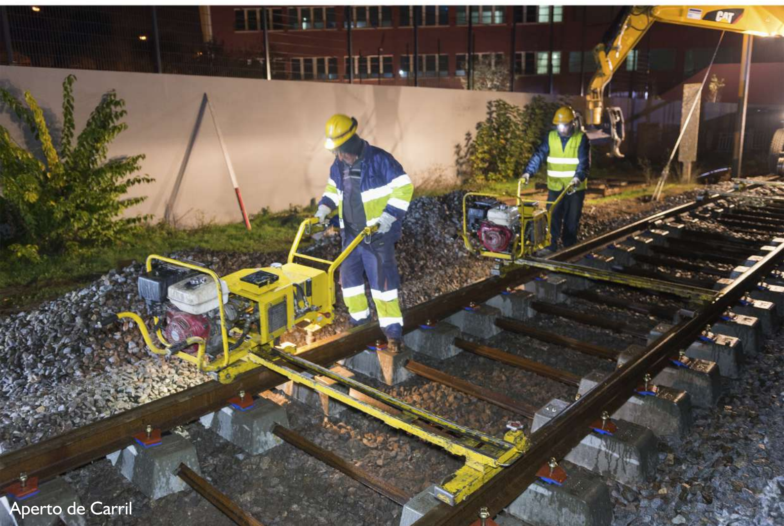
Preparação para Aperto de Carril
