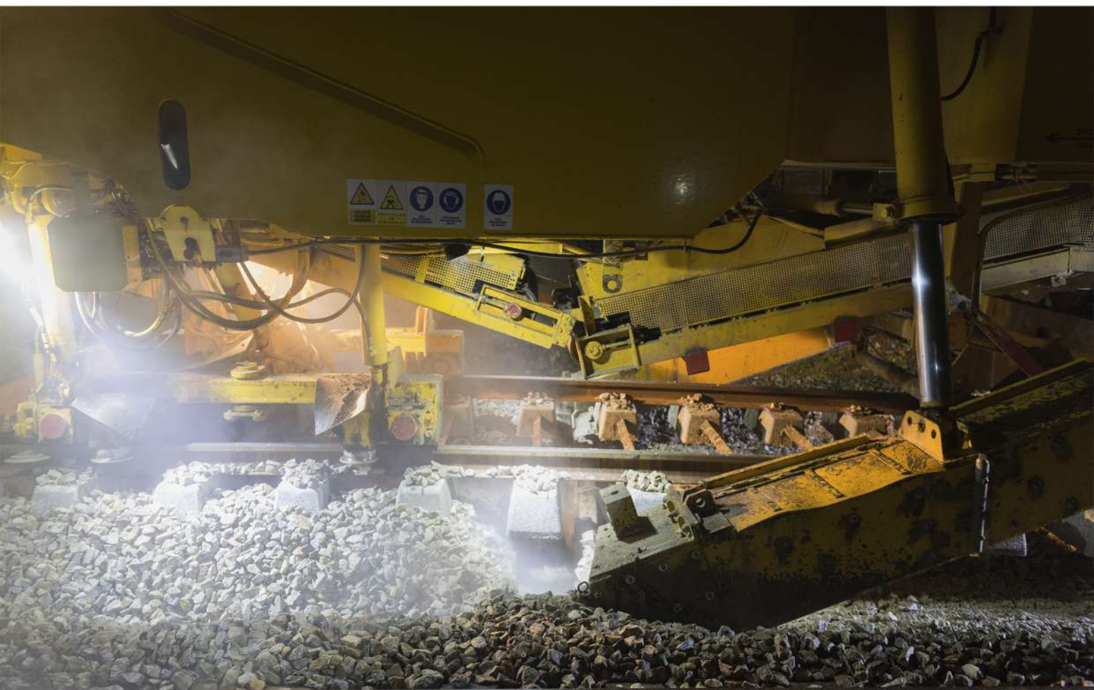
Desguarnecimento de Via
