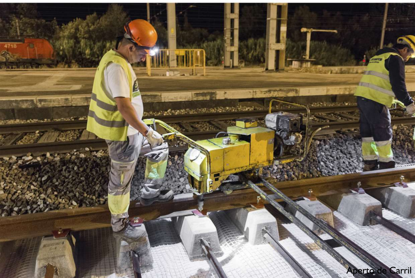
Renovação Integral de Via
