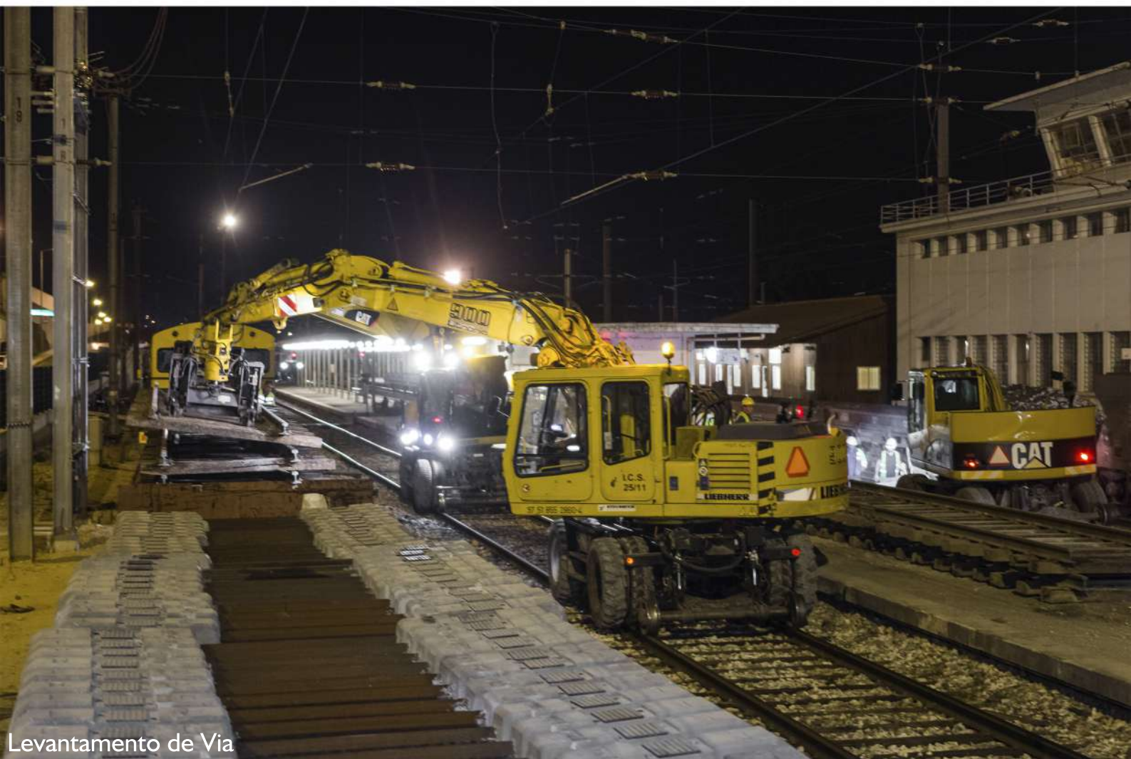
Levantamento de Via
