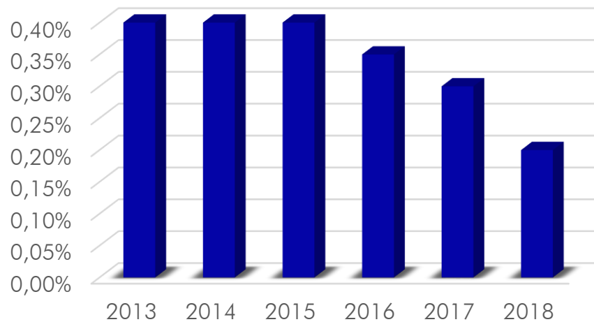
Verhältnis Q-Kosten vs. Umsätze (Ziel 2018: 0,20%)
