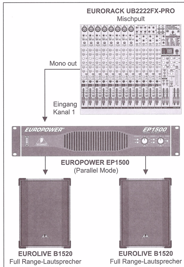
Abb. 3.3: Parallelbetrieb
