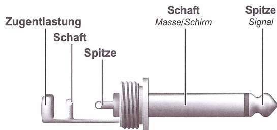
Abb. 4.4: 6,3-mm-Monoklinkenstecker
