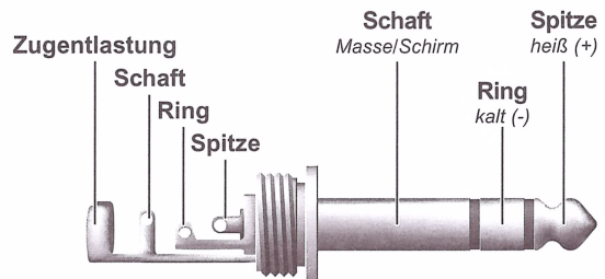
Abb. 4.5: 6,3-mm-Stereoklinkenstecker
