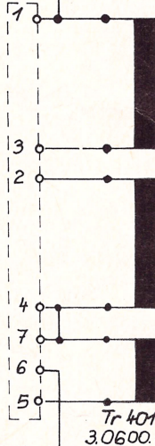
Spannungswahlschalter
